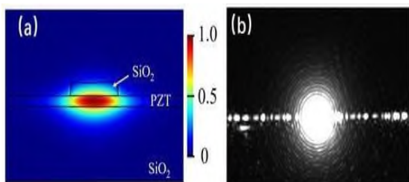
Сурет 4 – (a) толқындық модулятордағы модельденген оптикалық модель профилі; (b) CCD камерасы жинаған TE режимінің шығыс жарығы.
