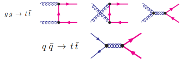
Сурет 2. t\bar{t} - кварктардың пайда болуын сипаттайтын диаграммалар.
